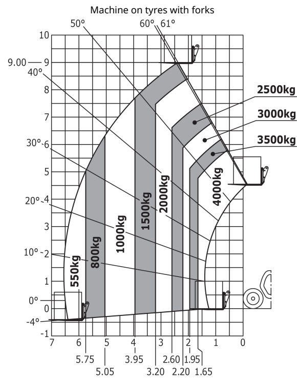
Rough terrain load chart (EN 1459 B)
