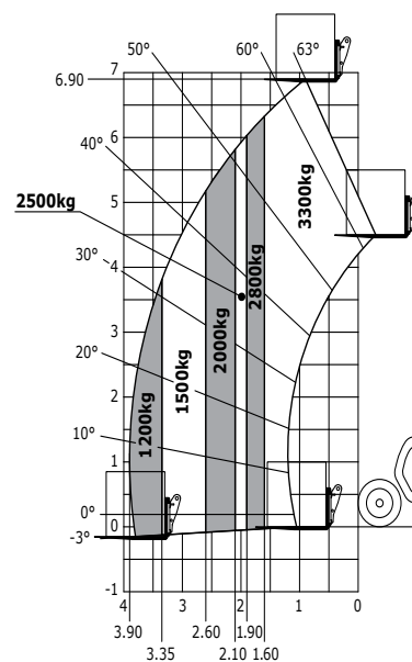
Maastokaavio (EN 1459 B)
