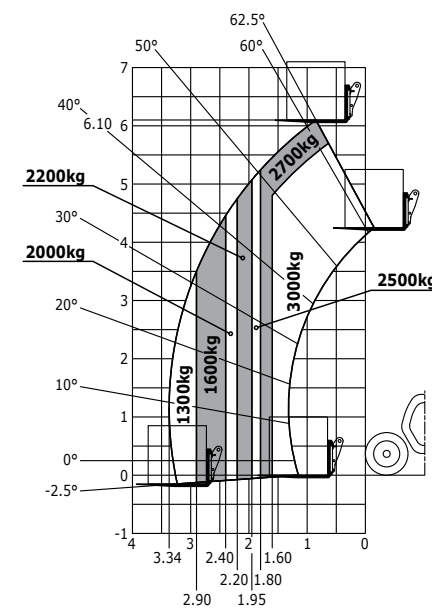
Maastokaavio (EN 1459 B)
