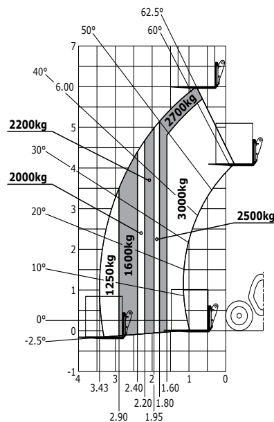
Maastokaavio (EN 1459 B)
