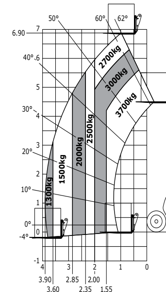
Maastokaavio (EN 1459 B)
